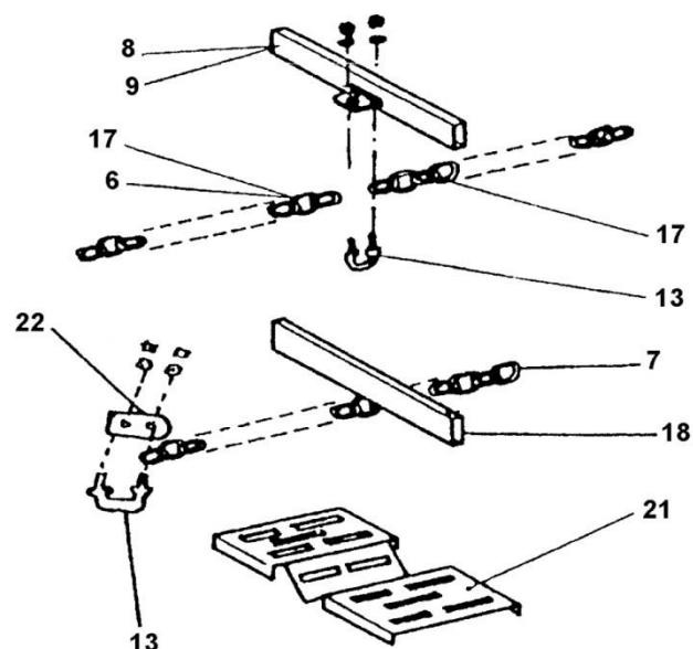
CHASSIS D'ANGLE, CHAINES ET RACLETTES GRILLES SUR PUISARD HOEKELEMENT, KETTINGEN, LATTEN ROOSTERS OP STERFPUT Ref. : 0A03400
