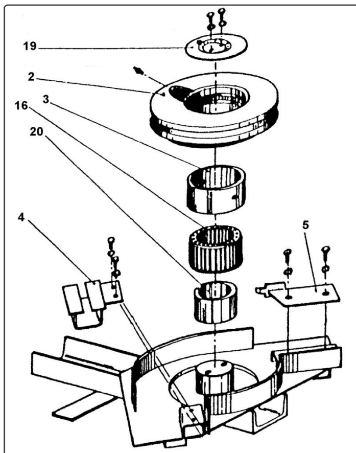
CHASSIS D'ANGLE, CHAINES ET RACLETTES GRILLES SUR PUISARD HOEKELEMENT, KETTINGEN, LATTEN ROOSTERS OP STERFPUT Ref. : 0A03400
